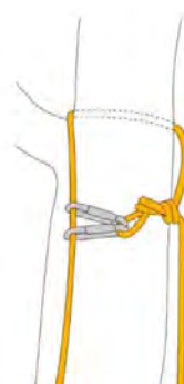
Fig. 3 - Possibile variante dello strozzo diretto della fune
