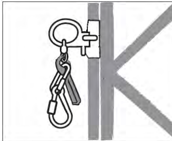
figura 7.1.1_1 dispositivo anticaduta di tipo guidato
