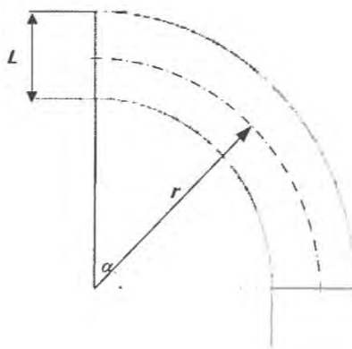
fig. 1 — rappresentazione schematica dei requisiti di curva minima
